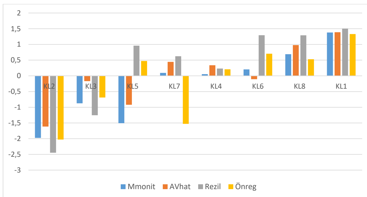
10.8. ábra. A PIK16 kérdőív 4 skáláján elvégzett MKA elemzés 9-klaszteres VEE8 megoldásában a z_t -standardizált átlagok oszlopdiagramja
