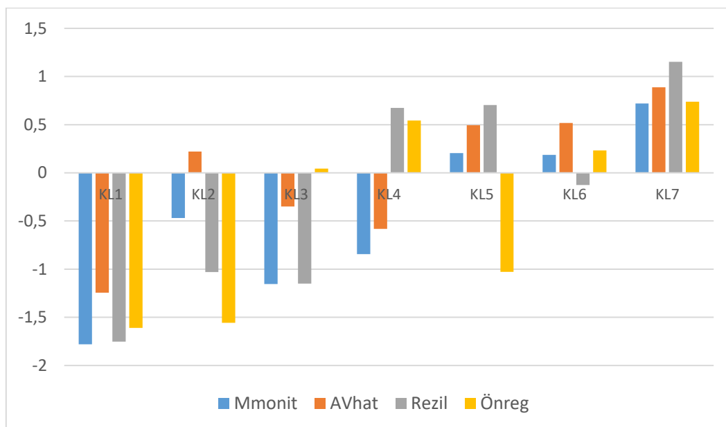
9.12. ábra. A 7-klasztteres k -közép megoldás z_i -standardizált átlagainak oszlopdiagramja
