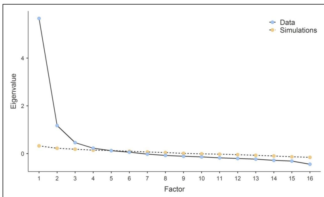
5.2. ábra. A PIK16 tételre alkalmazott EFA elemzés lejtődiagramja
